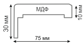
Наличник Телескоп Trim Telescope
