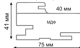
Коробка ПК 40 (41*75) Frame PC 40 (41*75)
