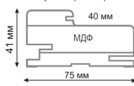
Добор Телескоп Transom Telescope
