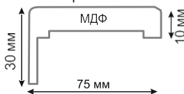
Наличник Телескоп Trim Telescope
