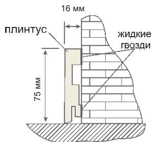
Крепление плинтуса на жидкие гвозди
