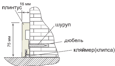
Крепление плинтуса с помощью кляймера(клипсы)
